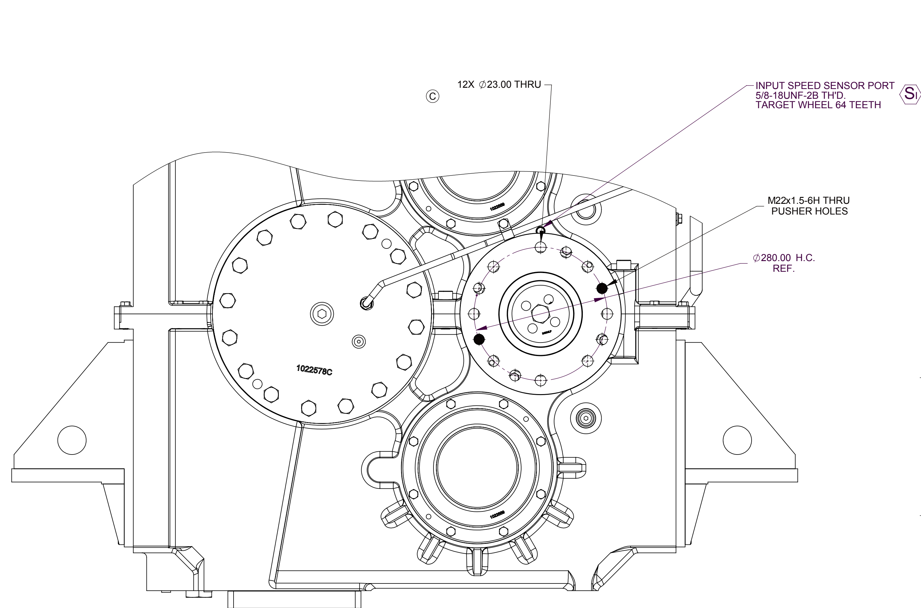
SECTION A-A
