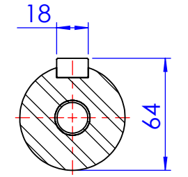
SEZIONE A-A
