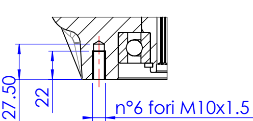
SEZIONE D-D
