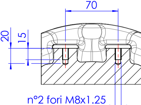
SEZIONE E-E
