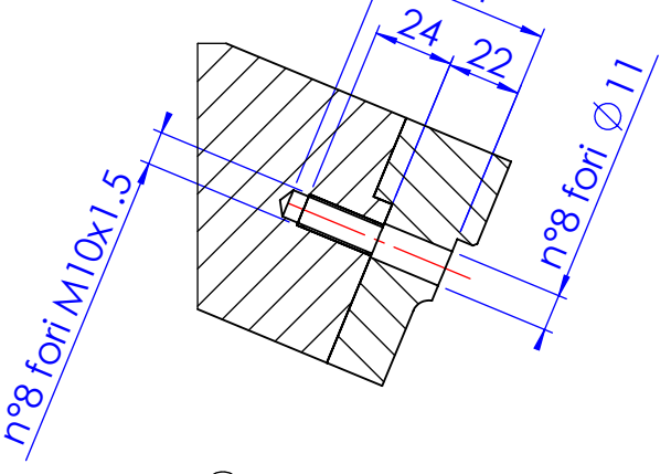
SEZIONE G-G
