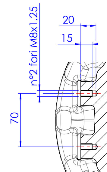
SEZIONE E-E
