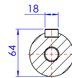
SEZIONE A-A
