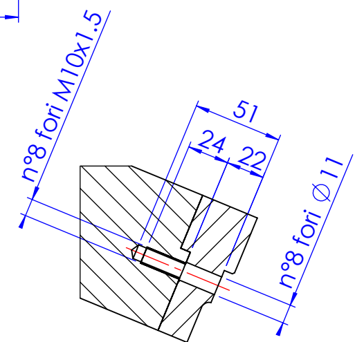
SEZIONE D-D
