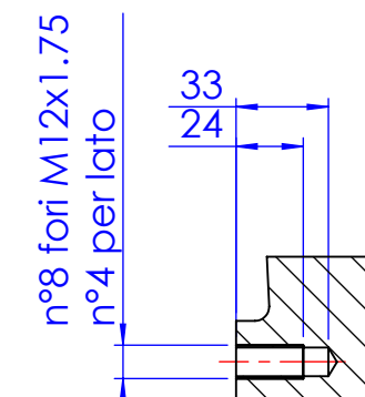
SEZIONE B-B
