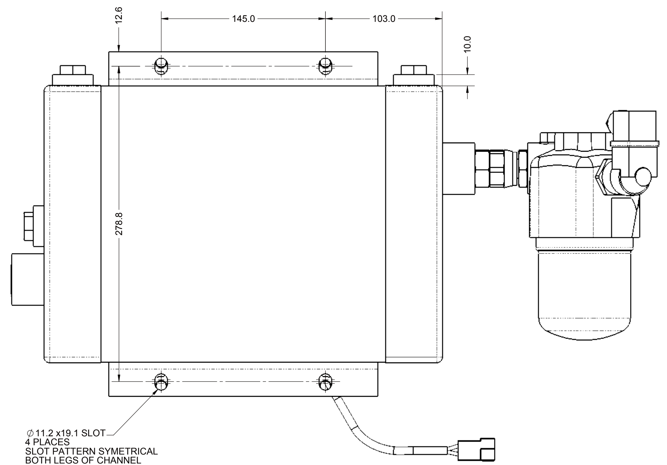
VIEW A-A
