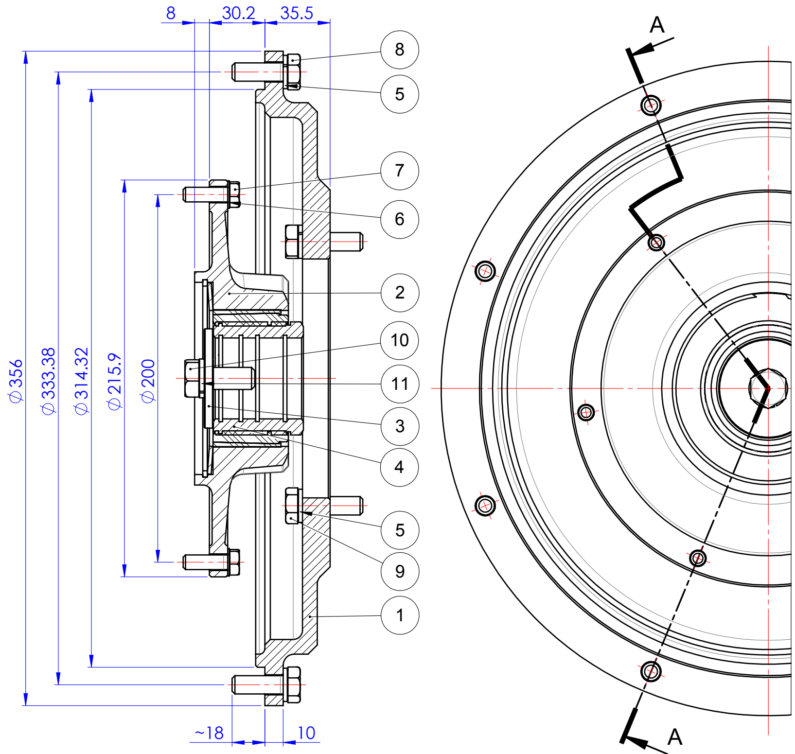
SEZIONE A-A
